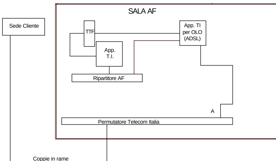
Figura 8- Co-locazione Virtuale con acquisto ed installazione dell'apparato a cura di Telecom Italia
