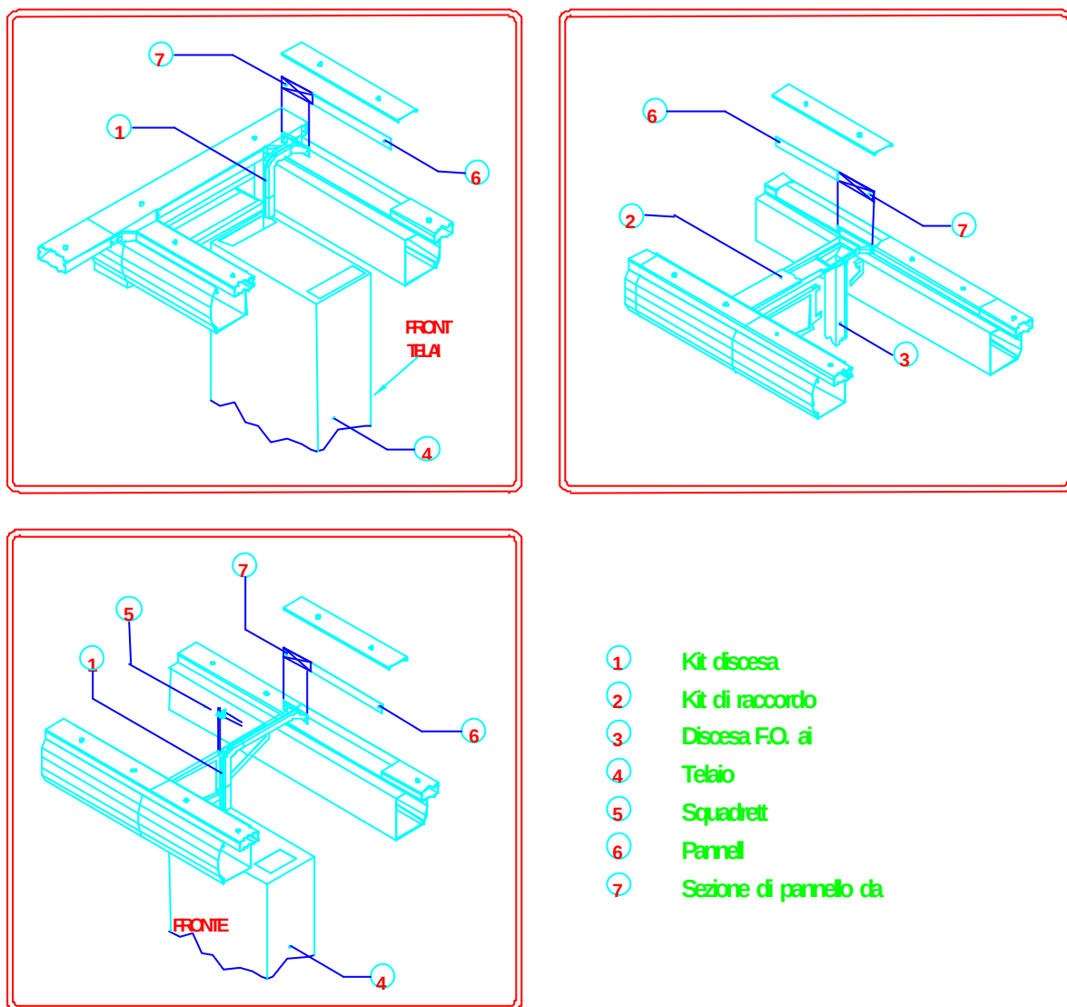
Figura 31: Esempio di canalizzazioni per discese f.o.
