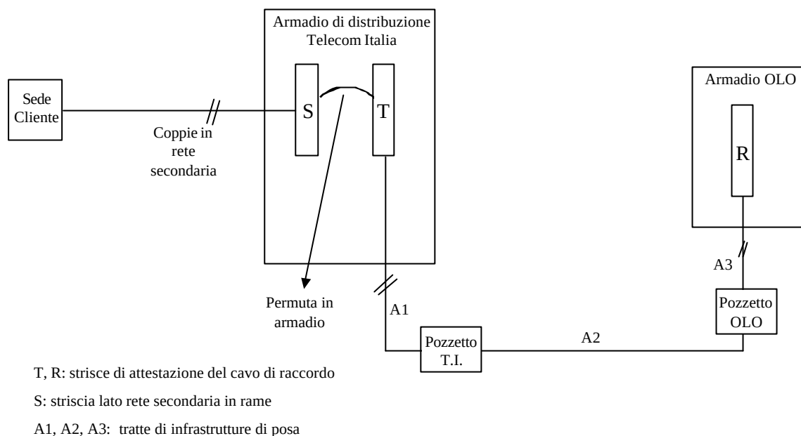
Figura 6- Co-locazione per servizi di accesso disaggregato alla sottorete locale
