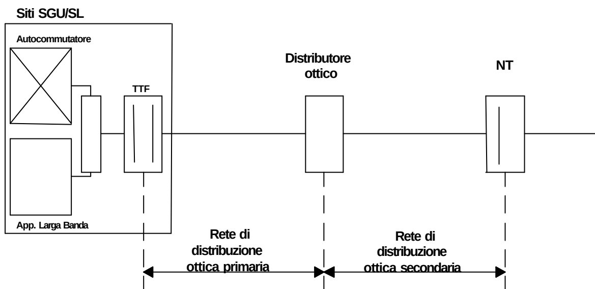
Figura 14-Rete di distribuzione in fibra ottica
