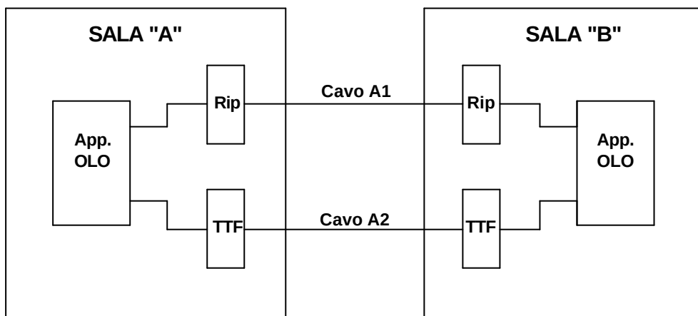
Figura 3 Raccordi per collegamento tra due sale Operatori
