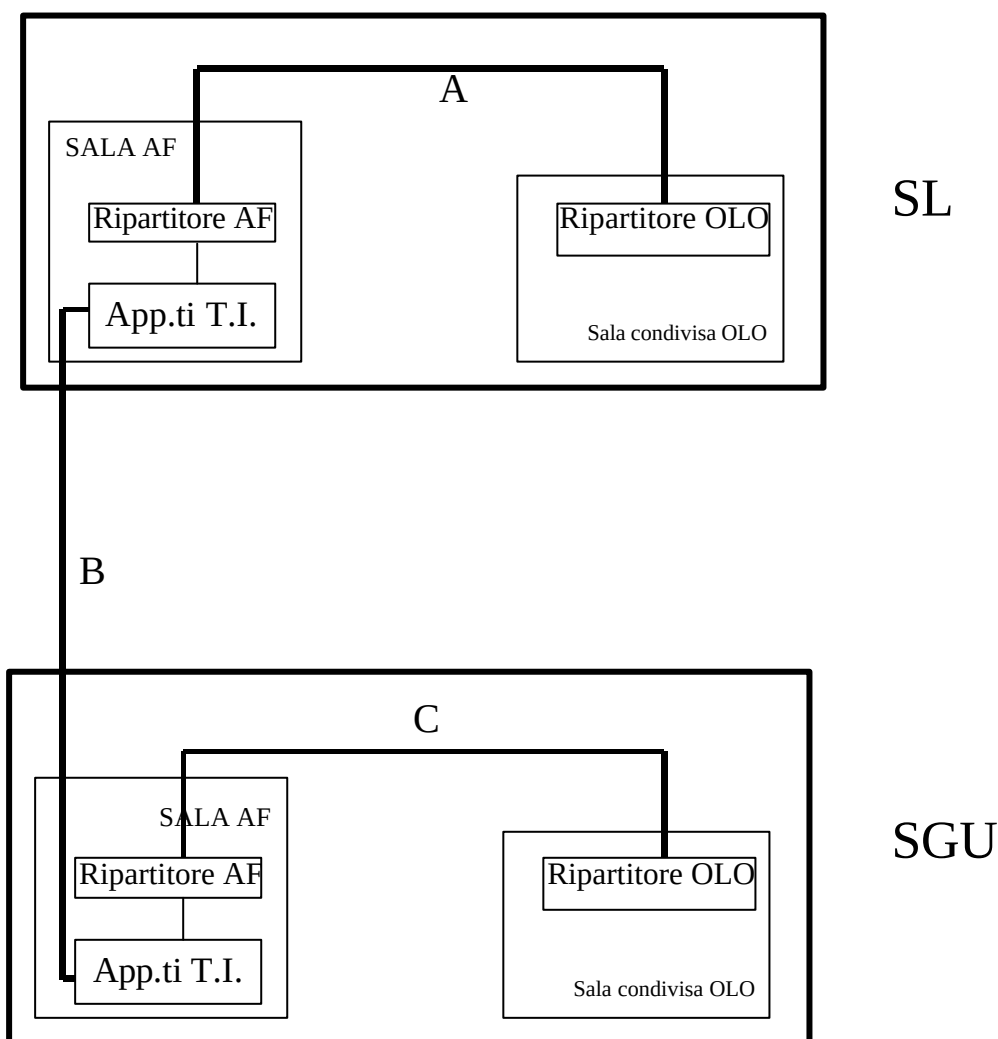
Figura 17 - Prolungamento dell'accesso SL-SGU con canale numerico
