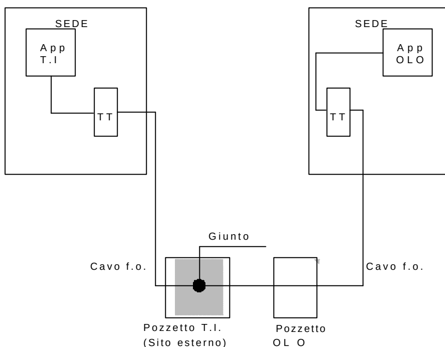
Figura 4 –Co-locazione in sito adiacente
