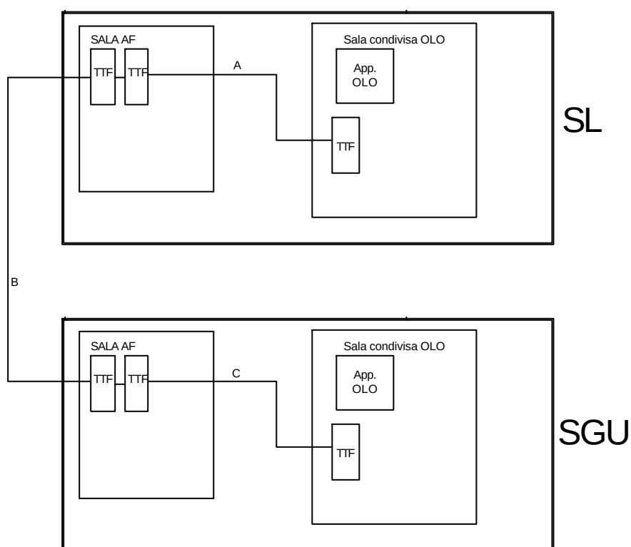
Figura 18 - Prolungamento dell'accesso SL-SGU su portante in fibra
