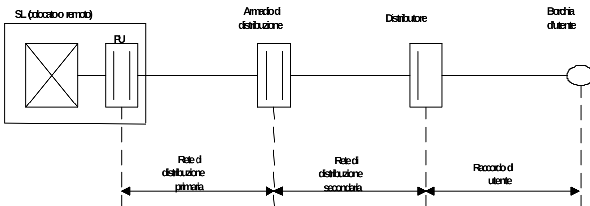
Figura 10 Rete di distribuzione in rame
