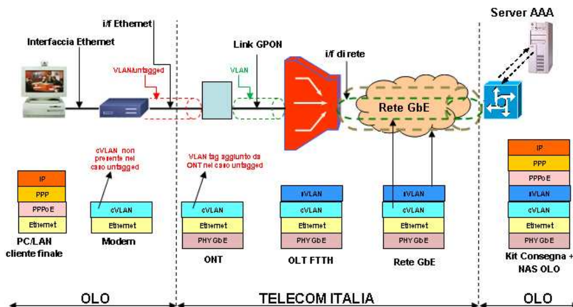
Figura 12: Protocollo PPPoE su accessi FTTH su banda “Double tag”
