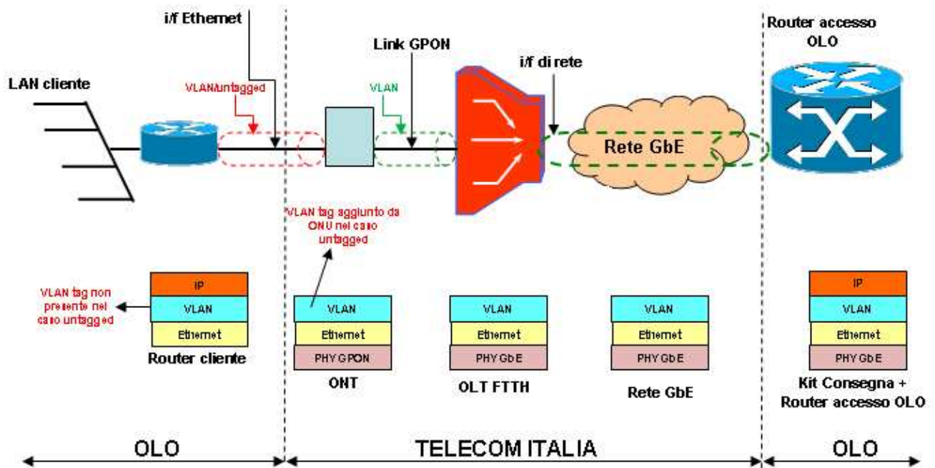
Figura 9: Protocollo IPoE su accessi FTTH su banda “Single tag”
