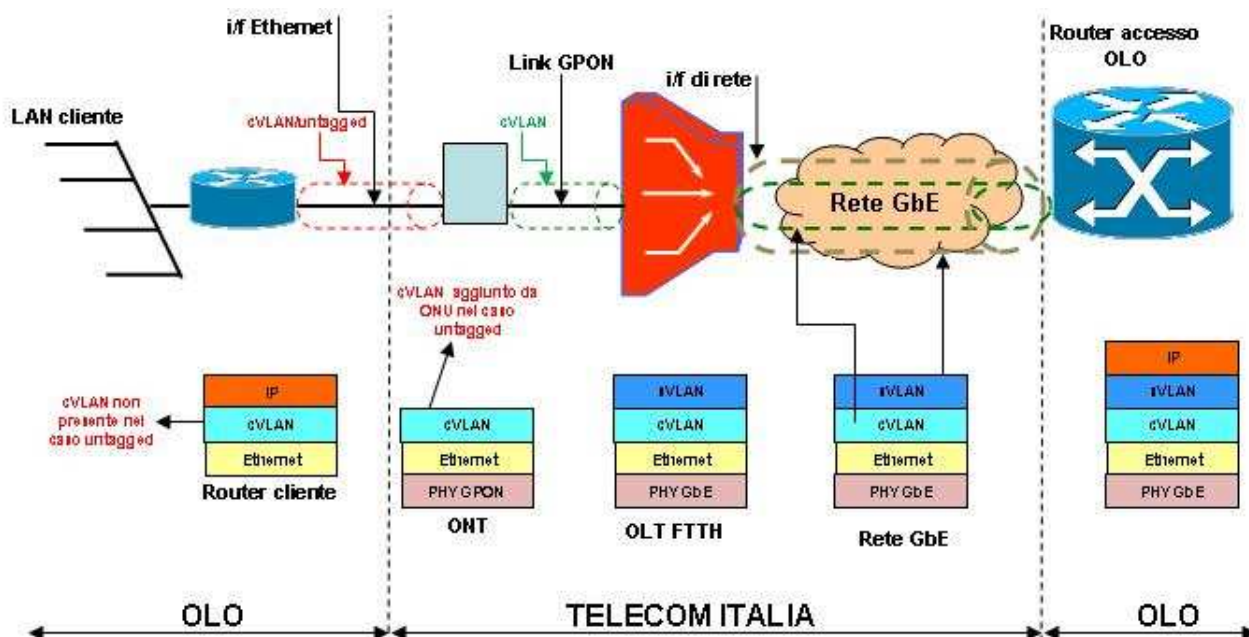
Figura 13: Protocollo IPoE su accessi FTTH su banda “Double tag”
