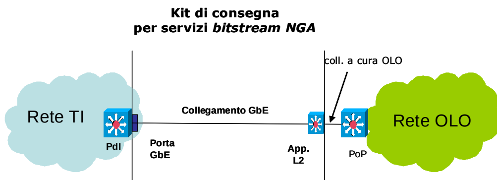
Figura 3: Kit di consegna Ethernet per servizi bitstream NGA.
