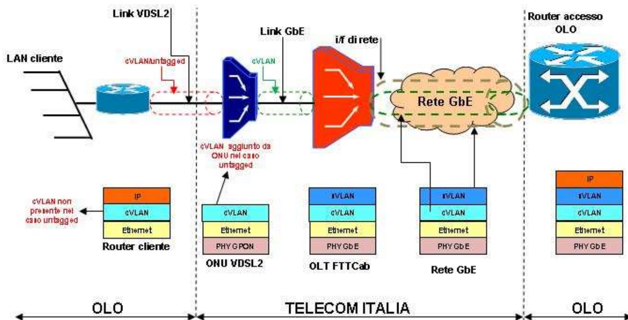
Figura 11: Protocollo IPoE su accessi FTTCab su banda “Double tag”
