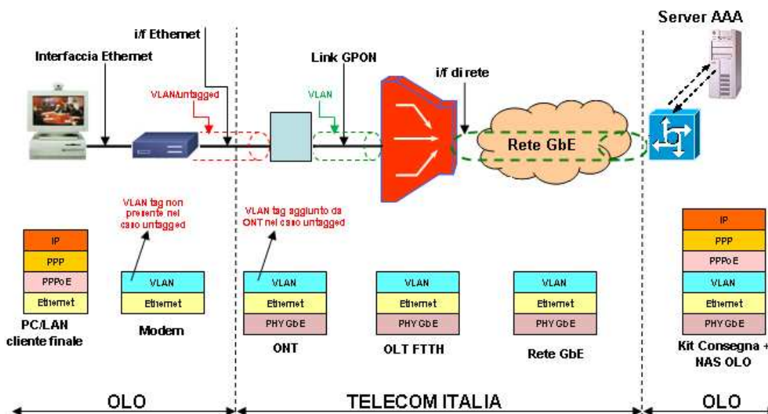
Figura 8: Protocollo PPPoE su accessi FTTH su banda "Single tag"
