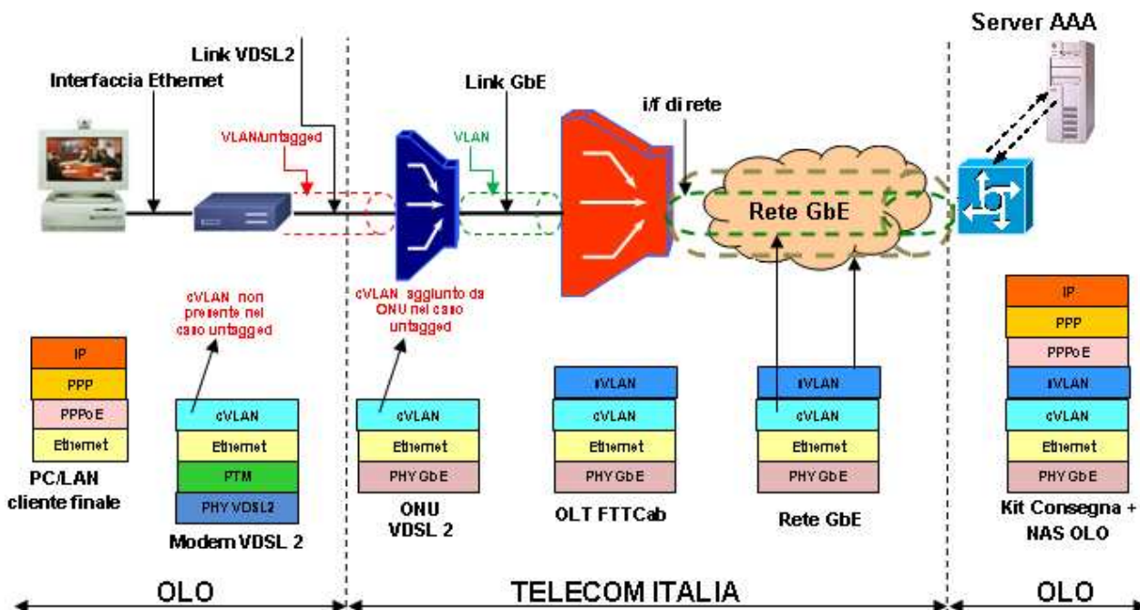
Figura 10: Protocollo PPPoE su accessi FTTCab su banda “Double tag”
