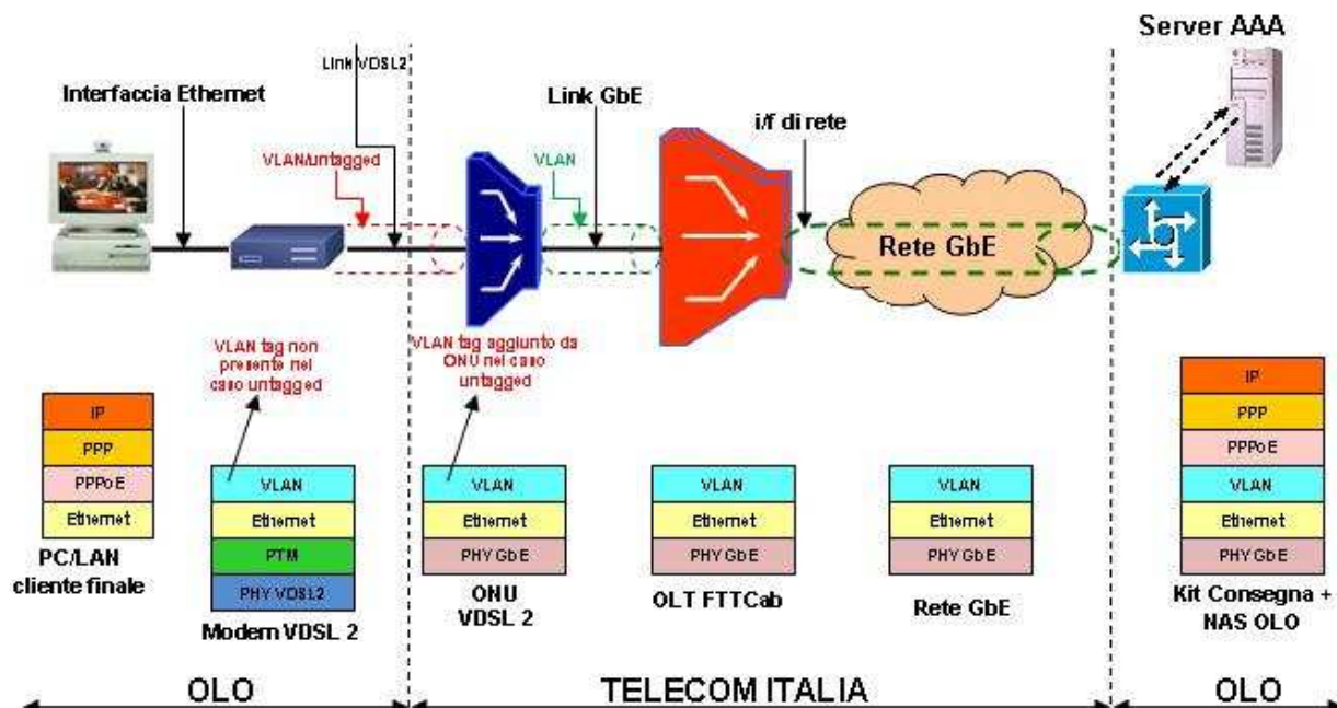
Figura 6: Protocollo PPPoE su accessi FTTCab su banda “Single tag”.
