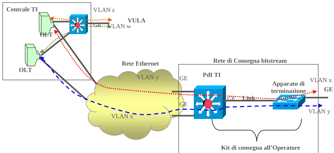
Figura 5: Architettura del trasporto e consegna della Banda Ethernet
