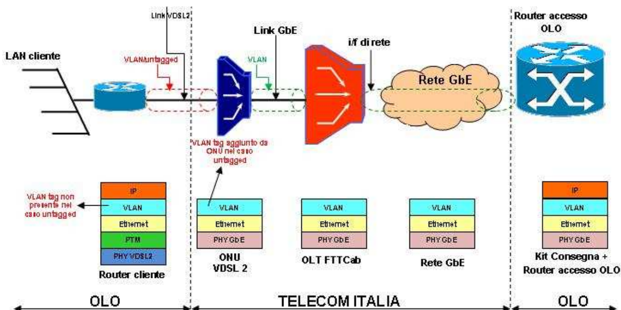
Figura 7: Protocollo IPoE su accessi FTTCab su banda “Single tag”
