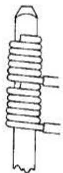
Figura 54: Esempio di doppia connessione sullo stesso terminale
