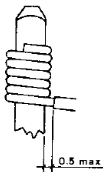
Figura 48: Distanza guaina dal terminale
