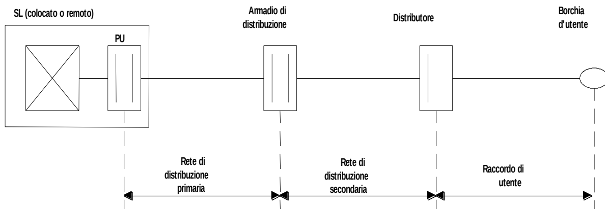
Figura 11: Rete di distribuzione in rame
