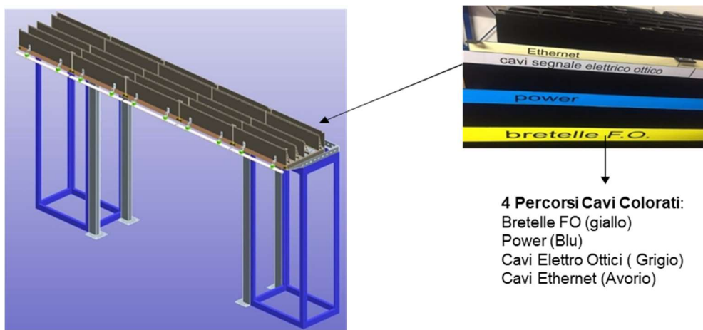
Figura 2 percorso cavi
