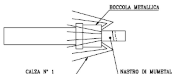
Figura 97 – Asportazione guaina e inserimento della boccola metallica
