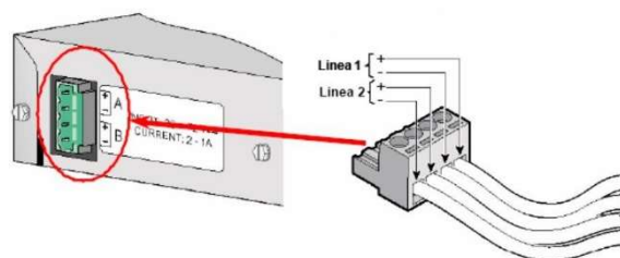
Figura 78 - Terminazione cavo unipolare su connettore di tipo plastico a morsettiera
