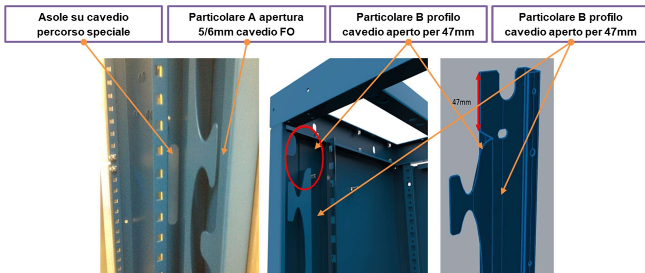
Figura 15 Particolari del Cavedio FO
