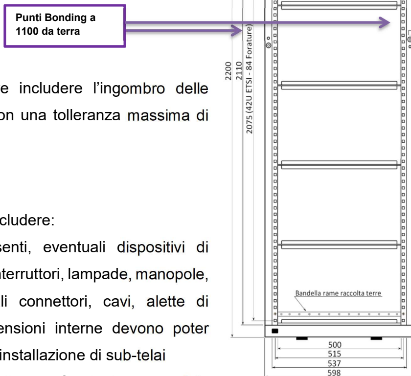
Figura 13 Struttura Base Telaio
