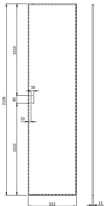
Figura 28 Portina Anteriore telaio
