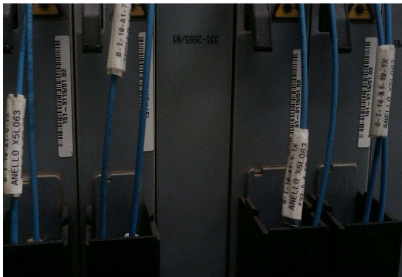
Figura 108 – Modalità di Etichettatura delle bretelle F.O.
