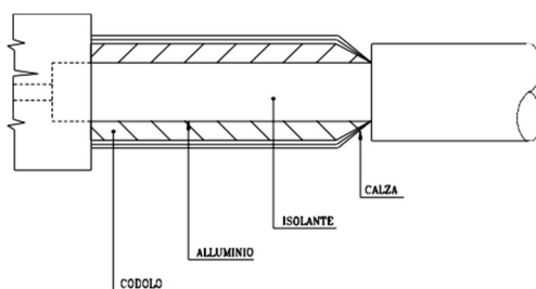
Figura 89 - Inserimento del cavo nel connettore
