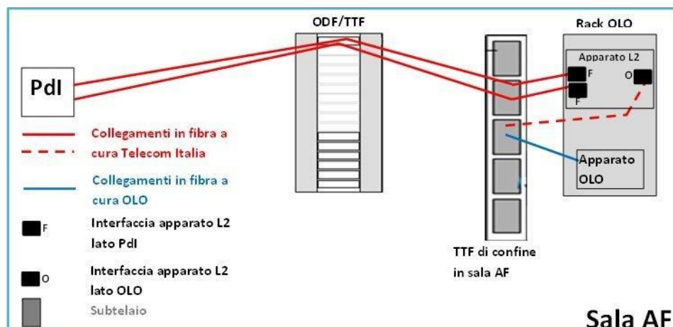
Figura 11 – Operatore in collocazione virtuale, Apparato L2 ospitato in spazi dell'Operatore
