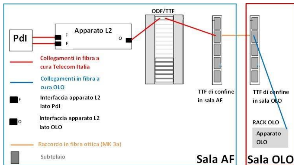
Figura 12 – Operatore in collocazione fisica, Apparato L2 ospitato in spazi Telecom Italia
