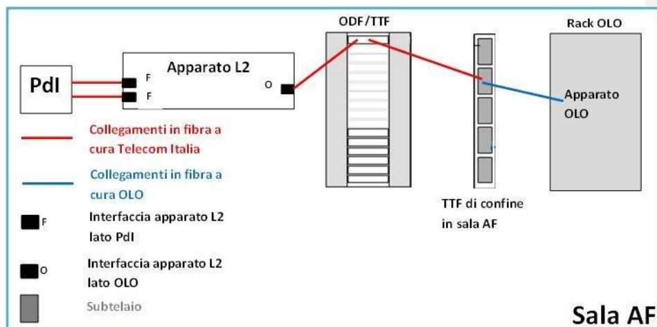
Figura 13 – Operatore in collocazione virtuale, Apparato L2 ospitato in spazi Telecom Italia
