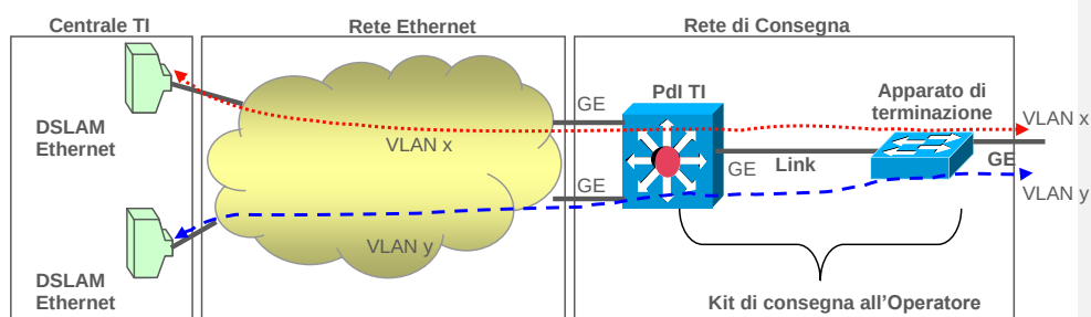
Figura 4: Architettura del trasporto Ethernet
