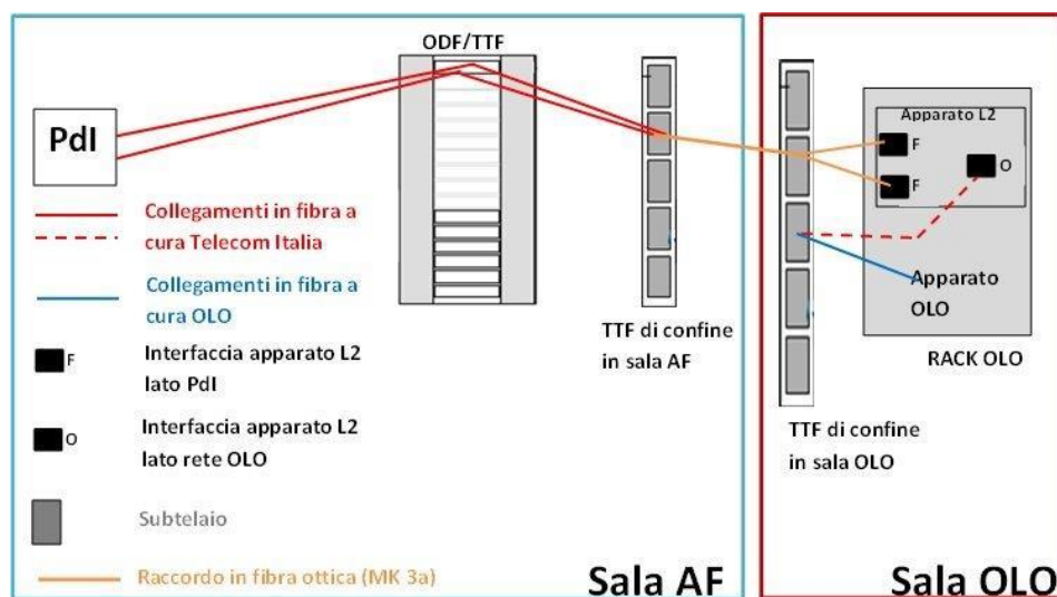
Figura 10 – Operatore in collocazione fisica, Apparato L2 ospitato in spazi dell'Operatore
