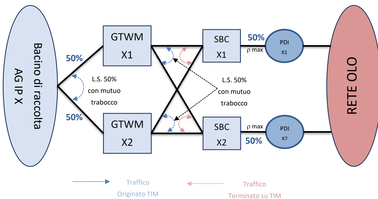
Figura 5: Criteri di Instradamento dei moduli CAC: attestazione a due Pdi
