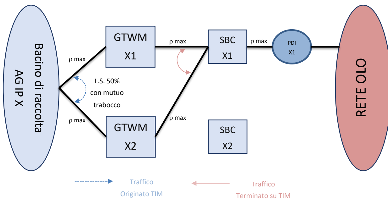
Figura 4: Criteri di dimensionamento dei moduli CAC: attestazione a Pdi singolo
