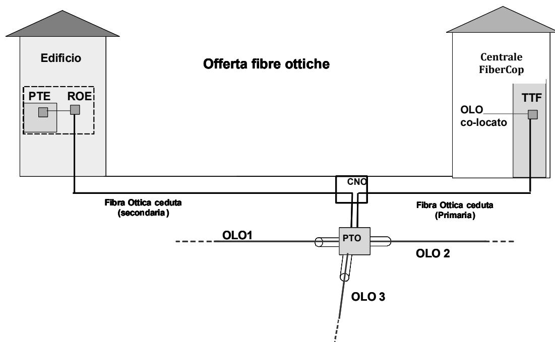
Figura 2: Rete Locale di Accesso in Fibra Ottica FTTH con architettura CNO
