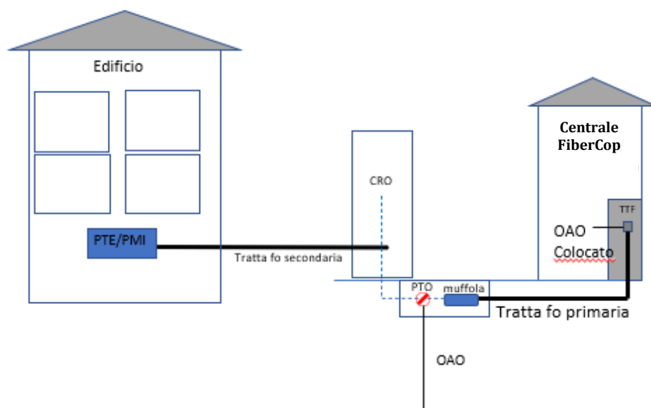
Figura 3: Rete Locale di Accesso in Fibra Ottica FTTH con architettura CRO
