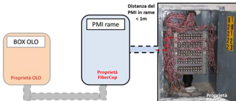
Figura 6: Schema operativo di massima per l'infrastruttura atta alla fornitura del Segmento di Terminazione in Rame
