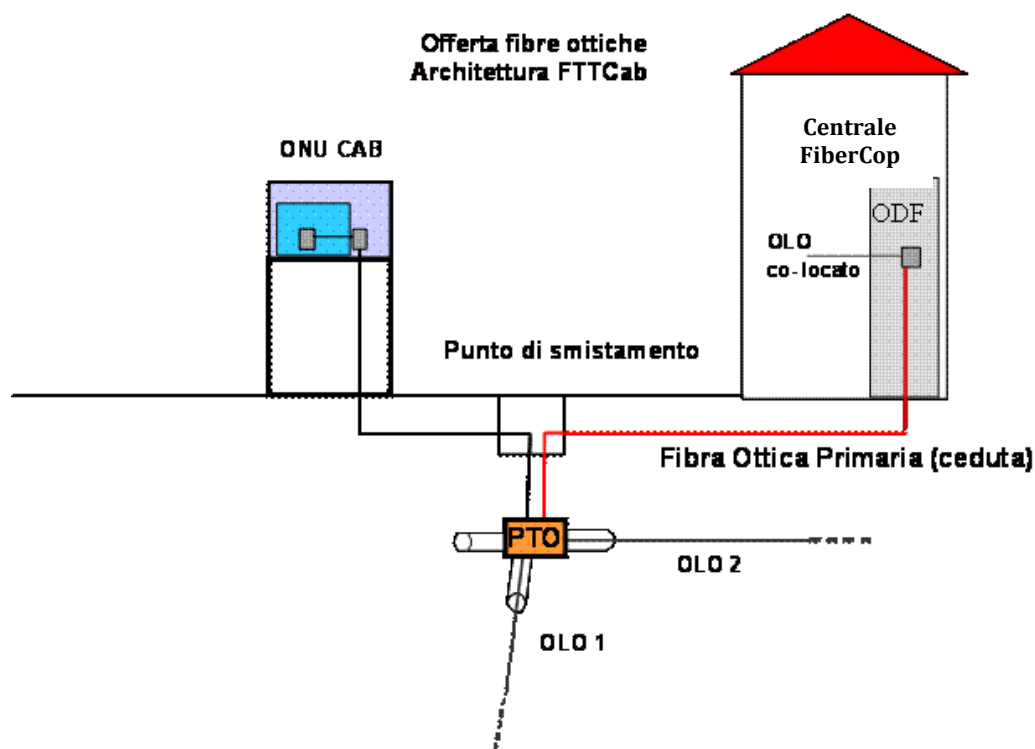
Figura 4: Rete Locale di Accesso in Fibra Ottica FTTCab
