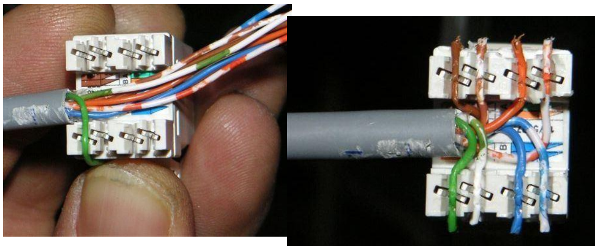
Figura 65 – Predisposizione dei conduttori su connettore femmina
