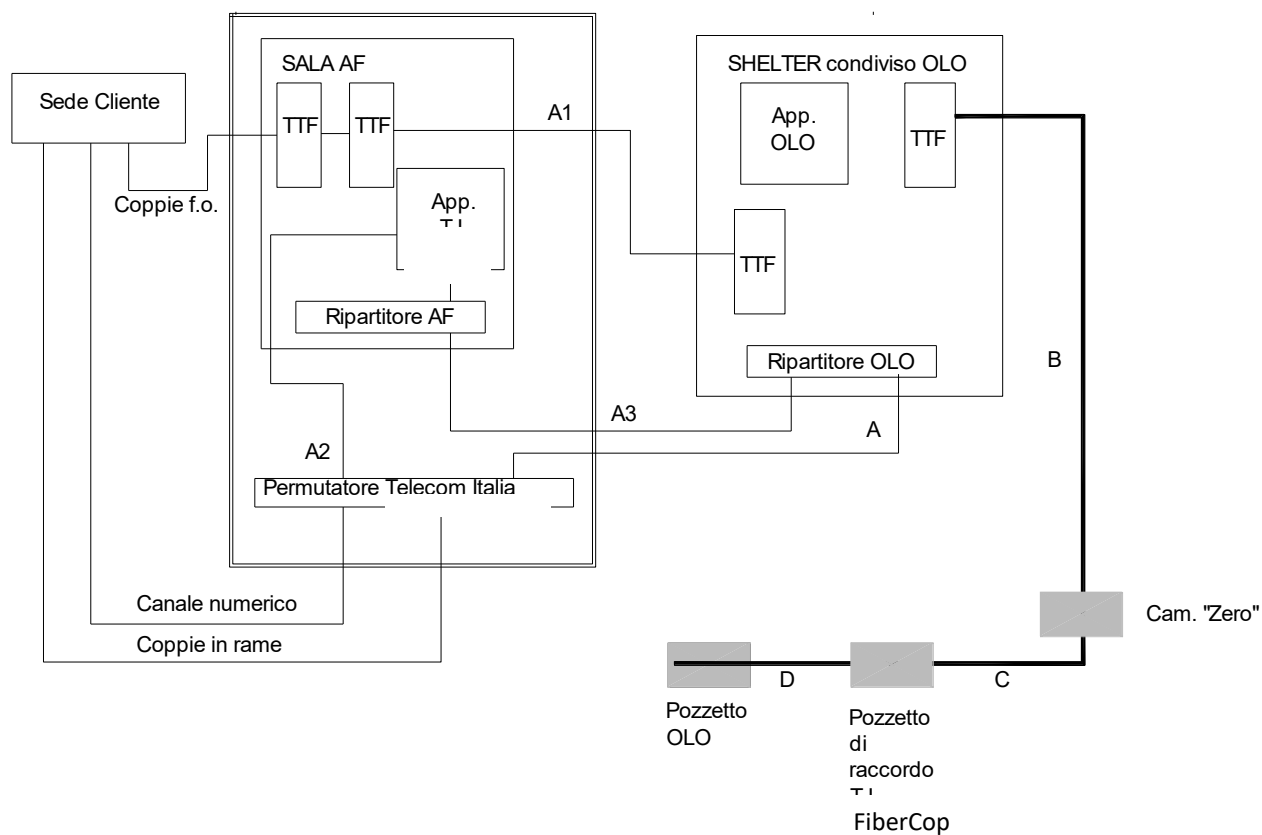
Figura 2: Colocazione Fisico B (esterno con shelter )
