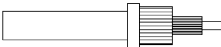
Figura 99 - Taglio a misura del conduttore centrale
