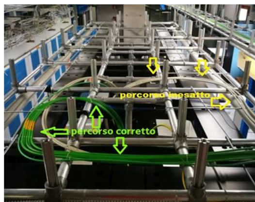
Figura 37 Esempio di posa cavo Breakout sul planare, percorso corretto (freccia verde)
