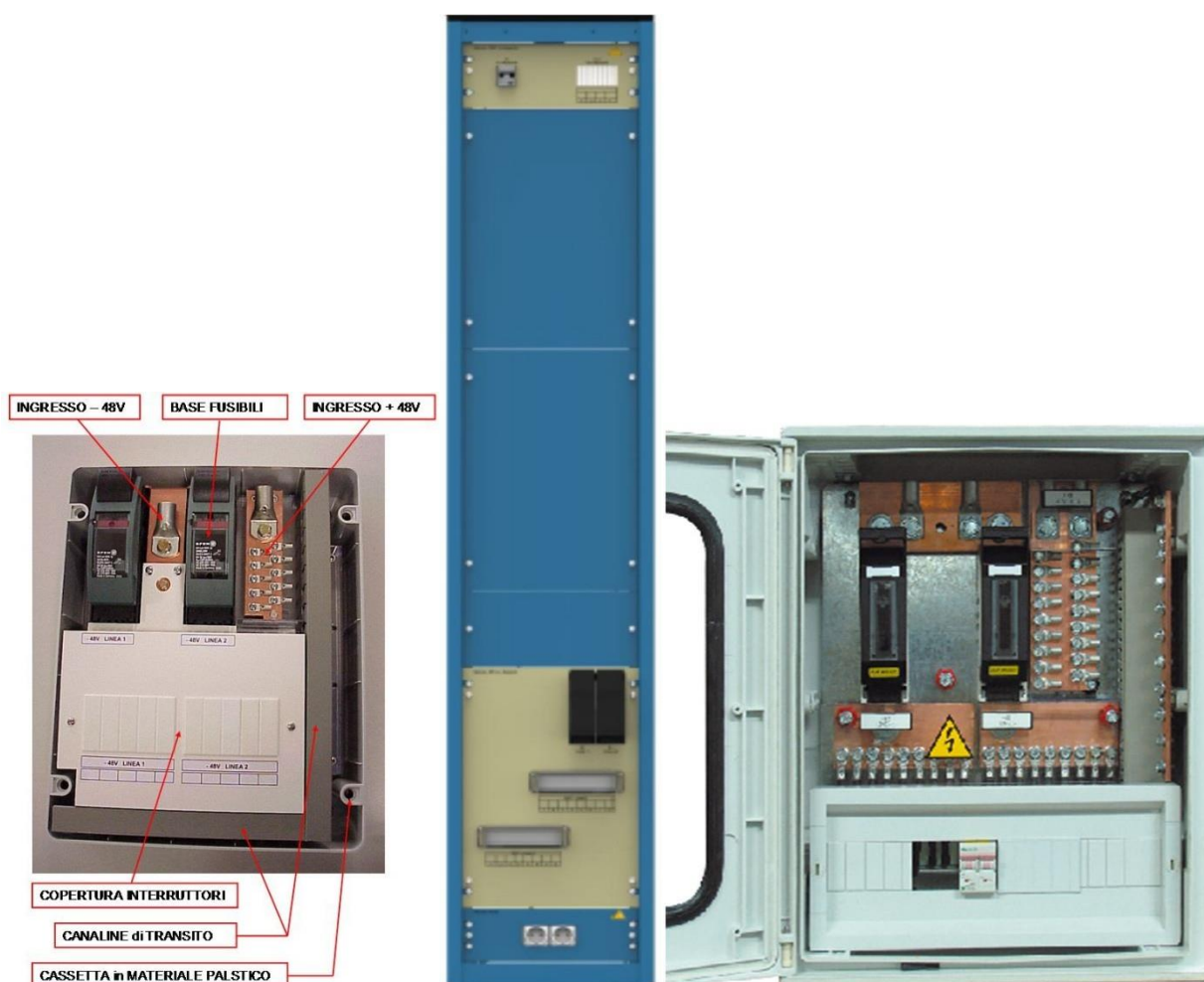
Figura 103 - Esempio di quadri esterni correntemente utilizzati
