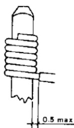
Figura 50 – Distanza guaina dal terminale
