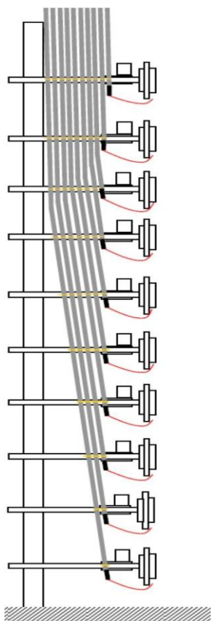
Figura 35 Esempio di posa su Ripartitore monofronte con un unico strato di cavi per tutti i livelli
