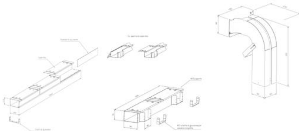
Figura 18 Canalina F.O. Alta potenzialità
