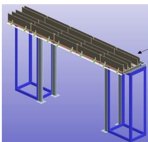
Figura 2 percorso cavi ST2016 versione I°
