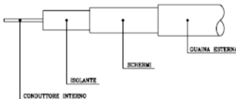
Figura 85 Disarmo del cavo
