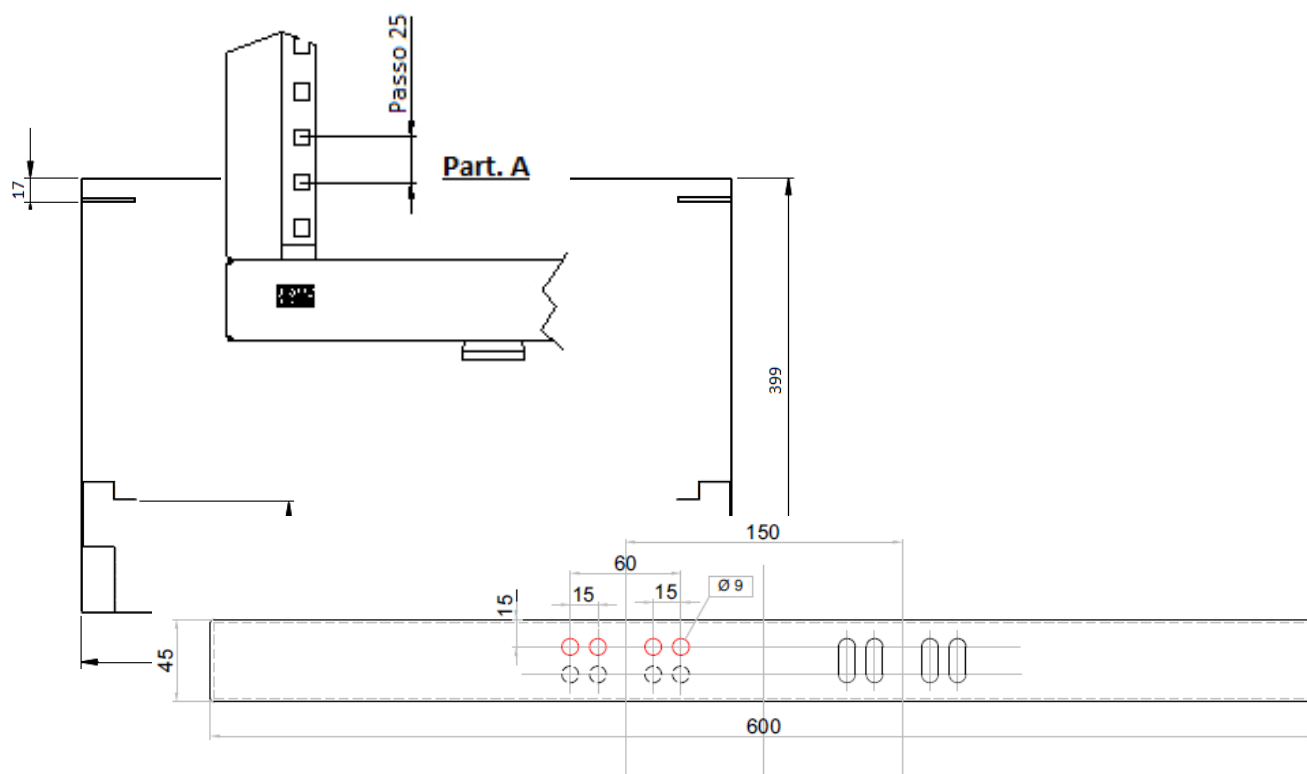
Figura 26 Piano posizionamento montanti ETSI
