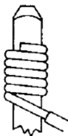
Figura 51 – Prima spira svolta
