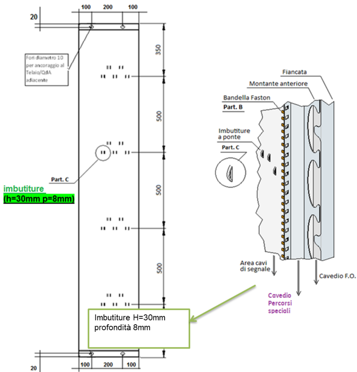
Figura 17 Fiancate Telaio
