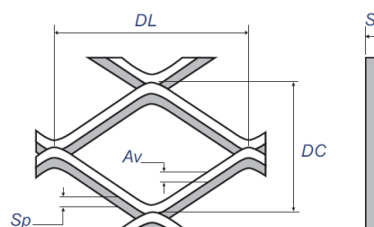
Figura 29 Caratteristiche lamiera portina Telaio
