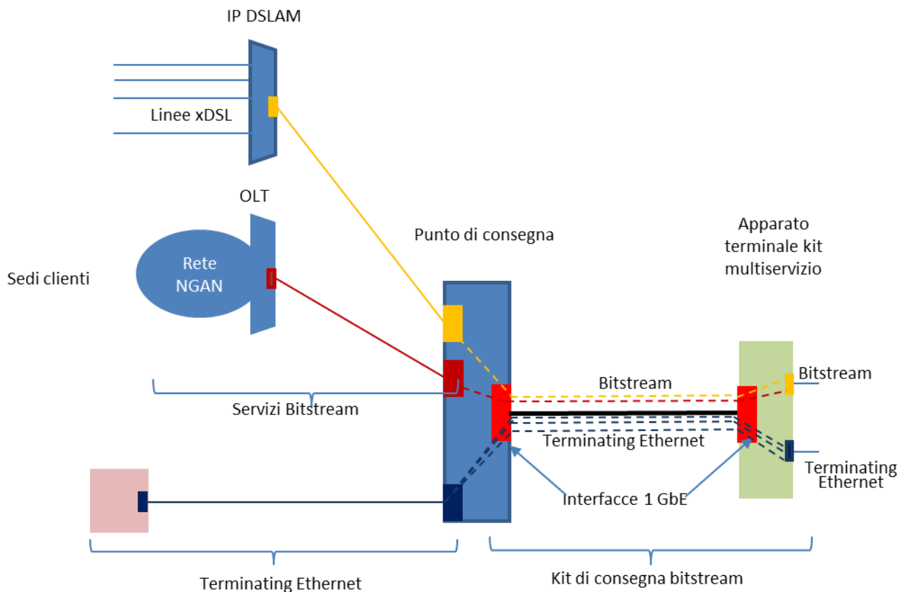
Figura 4: Raccolta circuito Terminating Ethernet su Kit Multiservizio
