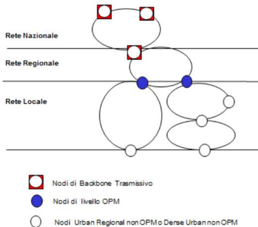
Figura 1: Architettura della rete trasmissiva di FiberCop
