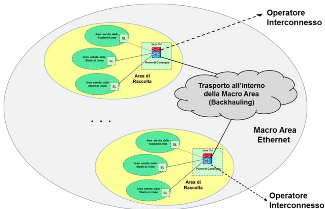
Figura 2: Macro Area Ethernet della rete di TIM
